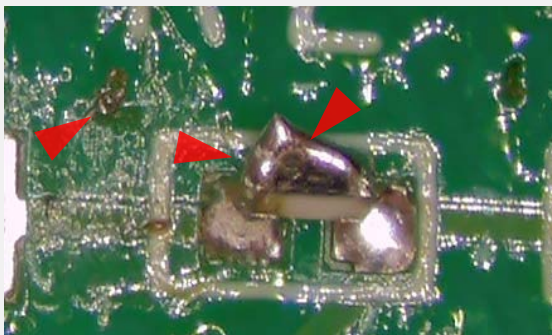
FOD&サイドのはみ出し IPC-A-610G 10.6.2, 8.3.2を参照
