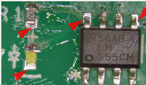
はんだ不足 IPC-A-610G 8.3.2, 8.3.5を参照
