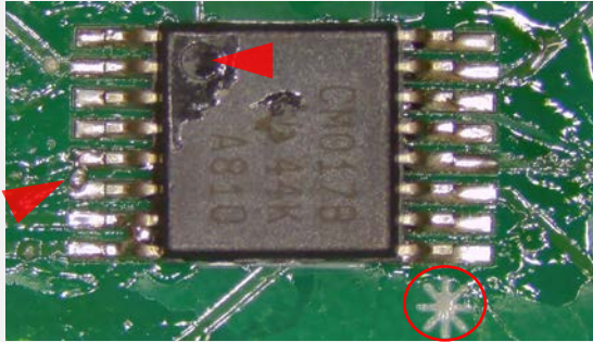
はんだブリッジ&取付方向相違 IPC-A-610G 5.2.7.2, 7.1.1.1を参照
