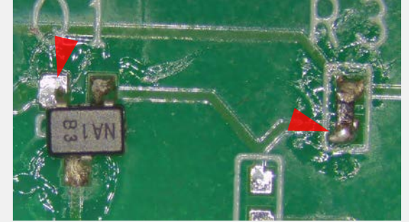
はんだ不足&はんだ過多 IPC-A-610G 8.3.5, 8.3.2を参照
