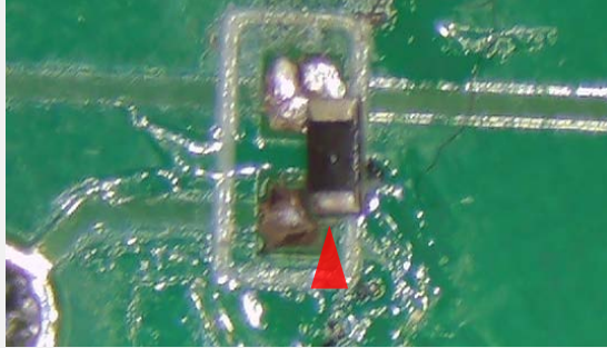
サイドのはみ出し IPC-A-610G 8.3.2を参照
