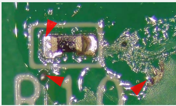
はんだ不足&はんだボール&FOD IPC-A-610G 8.3.2, 5.2.7.1, 10.6.2を参照
