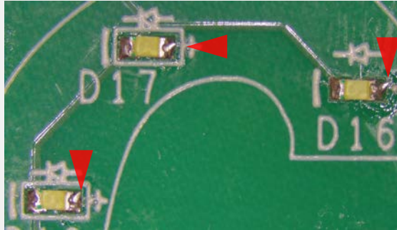
はんだの突起 IPC-A-610G 5.2.10を参照
