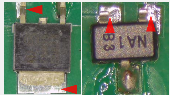
はんだ不足 IPC-A-610G 8.3.14, 8.3.5を参照
