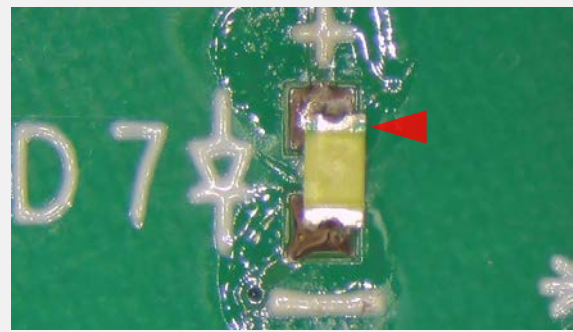
取付方向相違 IPC-A-610G 7.1.1.1を参照
