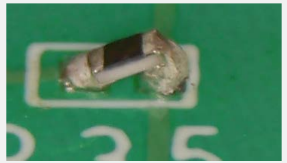
部品の浮き IPC-A-610G 8.3.2を参照
