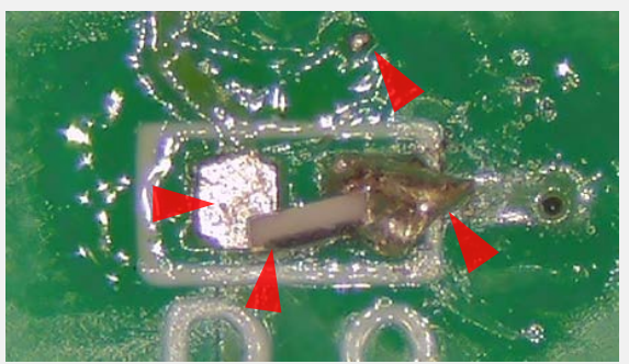
はんだ不足&部品の横転 IPC-A-610G 8.3.2, 8.3.2.9.1を参照
