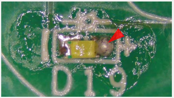
はんだ過多 IPC-A-610G 8.3.2を参照
