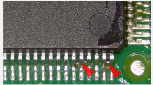
はんだブリッジ IPC-A-610G 5.2.7.2を参照
