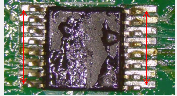
リード サイドのはみ出し IPC-A-610G 8.3.5を参照
