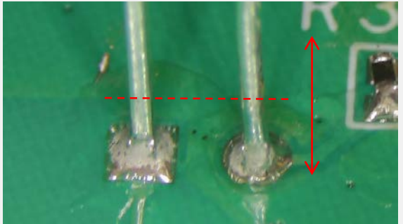
リードの突出 (最大値以上) IPC-A-610G 7.3.3を参照
