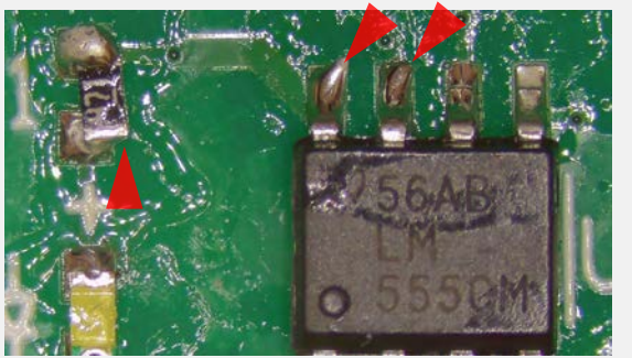
サイドのはみ出し&はんだの突起 IPC-A-610G 8.3.2, 5.2.10を参照
