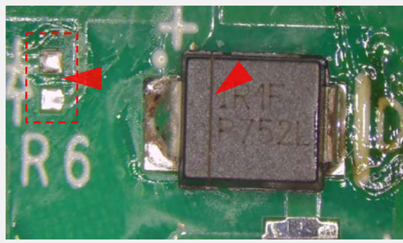
未取付&取付方向相違 IPC-A-610G 7.1.1.1を参照
