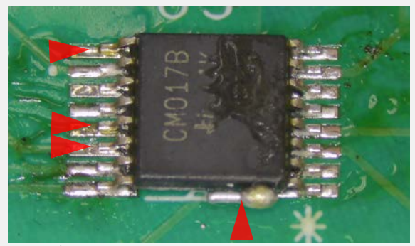
はんだ不足&FOD IPC-A-610G 8.3.5, 10.6.2を参照
