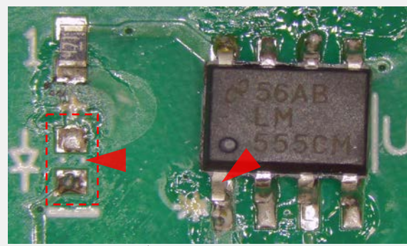
未取付&はんだ不足 IPC-A-610G 7.1.1.1, 8.3.5を参照
