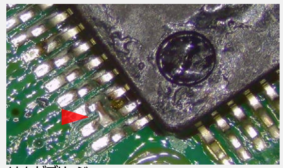
はんだブリッジ IPC-A-610G 5.2.7.2を参照
