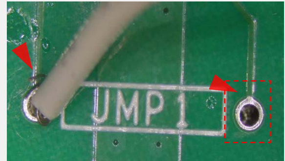
より線のほつれ&取付不完全 IPC-A-610G 6.3.4, 7.1.1.1を参照
