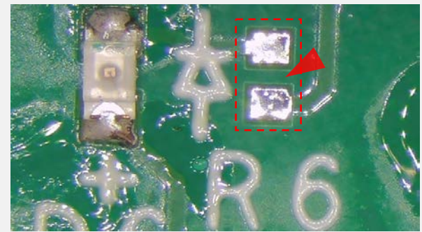
未取付 IPC-A-610G 7.1.1.1を参照
