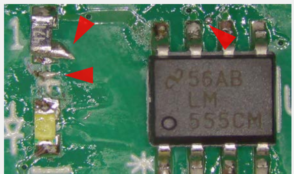
はんだの突起&FOD&はんだボール IPC-A-610G 5.2.10,10.6.2,5.2.7.1を参照
