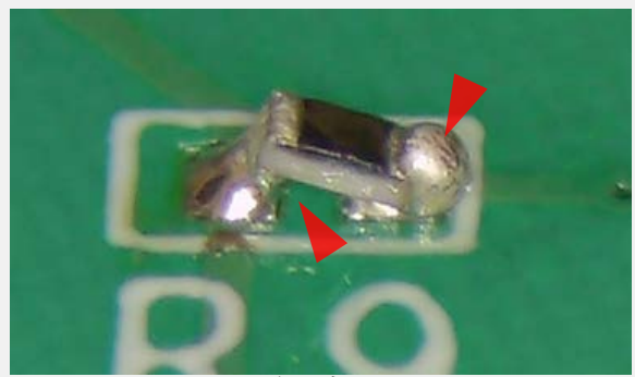
部品の浮き&はんだ過多 IPC-A-610G 8.3.2を参照
