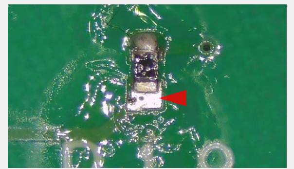
はんだ不足 IPC-A-610G 8.3.2を参照
