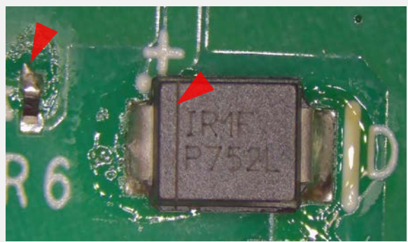
はんだの突起&取付方向相違 IPC-A-610G 5.2.10, 7.1.1.1を参照
