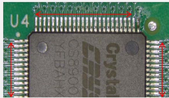
はんだ不足 IPC-A-610G 8.3.5を参照
