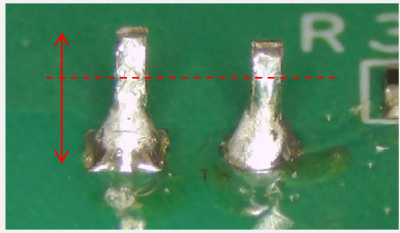
リードの突出 (最大値以上) IPC-A-610G 7.3.3を参照
