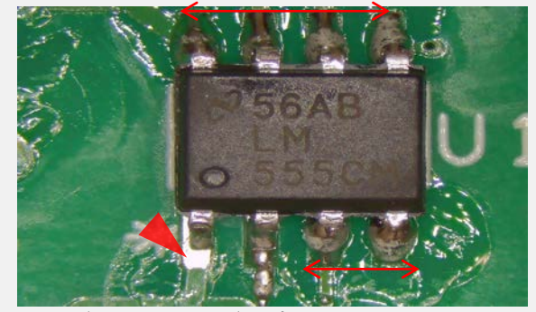
はんだ不足&はんだ過多 IPC-A-610G 8.3.5を参照
