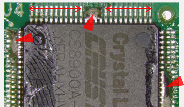
はんだブリッジ&はんだ不足 IPC-A-610G 5.2.7.2, 8.3.5を参照
