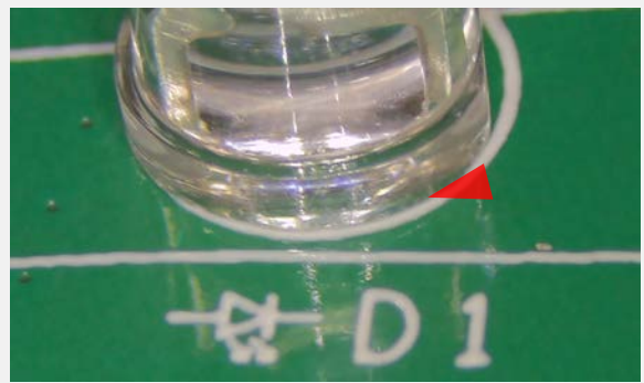
ラジアルリード垂直方向 クリアランス不足 IPC-A-610G 7.1.6を参照
