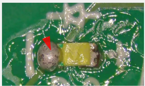
はんだ過多 IPC-A-610G 8.3.2を参照
