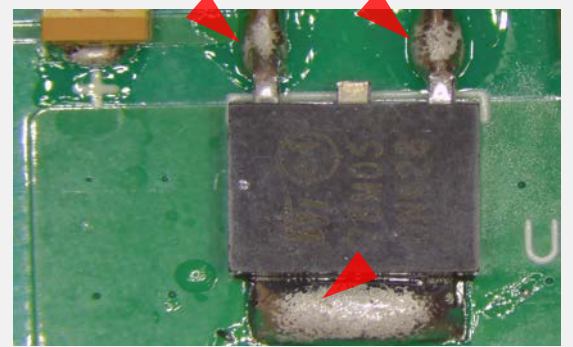
はんだ過多 IPC-A-610G 8.3.14を参照
