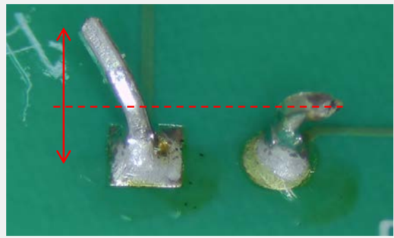
リードの突出 (最大値以上) IPC-A-610G 7.3.3を参照
