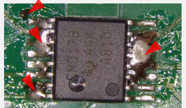
はんだブリッジ&FOD IPC-A-610G 5.2.7.2, 10.6.2を参照
