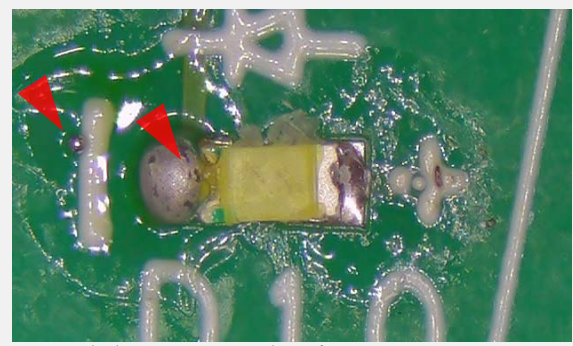
はんだボール&はんだ過多 IPC-A-610G 5.2.7.1, 8.3.2を参照
