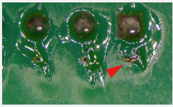
FOD IPC-A-610G 10.6.2を参照
