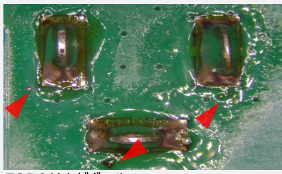
FOD&はんだボール IPC-A-610G 10.6.2, 5.2.7.1を参照
