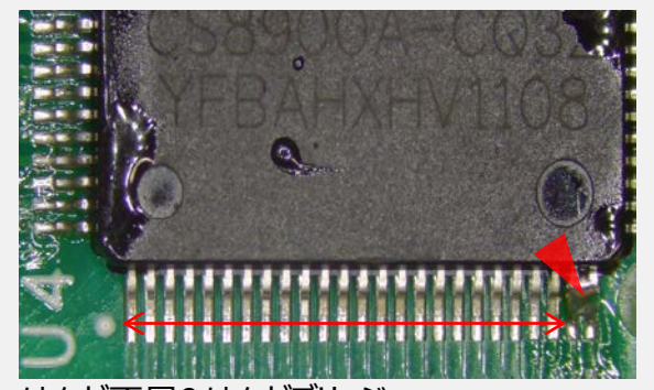
はんだ不足&はんだブリッジ IPC-A-610G 8.3.5, 5.2.7.2を参照
