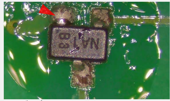
はんだ過多 IPC-A-610G 8.3.5を参照
