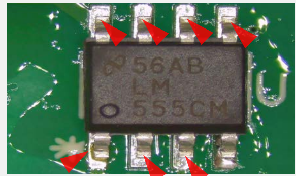
はんだ不足 IPC-A-610G 8.3.5を参照
