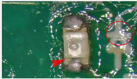
取付方向相違 IPC-A-610G 7.1.1.1を参照
