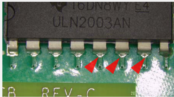
リードとスルーホール間のはんだのぬれ不足 IPC-A-610G 7.3.5を参照
