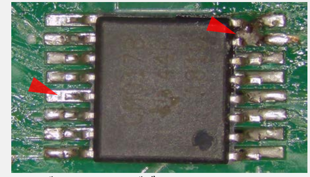
はんだ不足 & はんだブリッジ IPC-A-610G 8.3.5, 5.2.7.2を参照
