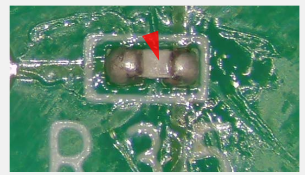
部品の表裏反転 IPC-A-610G 8.3.2.9.2を参照
