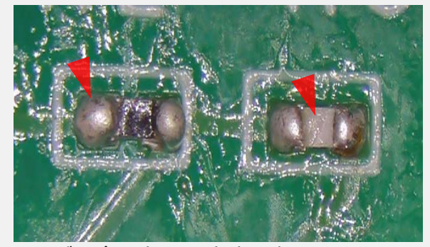
はんだ過多 & 部品の表裏反転 IPC-A-610G 8.3.2, 8.3.2.9.2を参照
