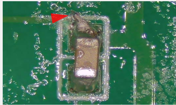
はんだの突起 IPC-A-610G 5.2.10を参照
