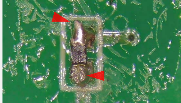
はんだの突起 & コールドはんだ接合 IPC-A-610G 5.2.10, 5.2.5を参照
