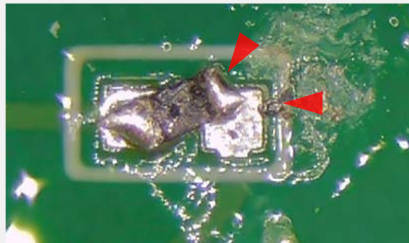
サイドのはみ出し&FOD IPC-A-610G 8.3.2, 10.6.2を参照
