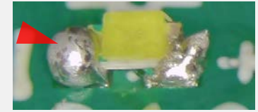
はんだ過多 IPC-A-610G 8.3.2を参照
