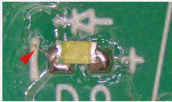
はんだウェビング／飛散 IPC-A-610G 5.2.7.3を参照
