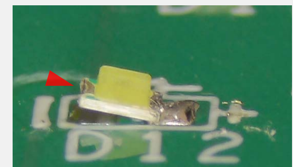
ツームストーン現象 IPC-A-610G 8.3.2.9.4を参照
