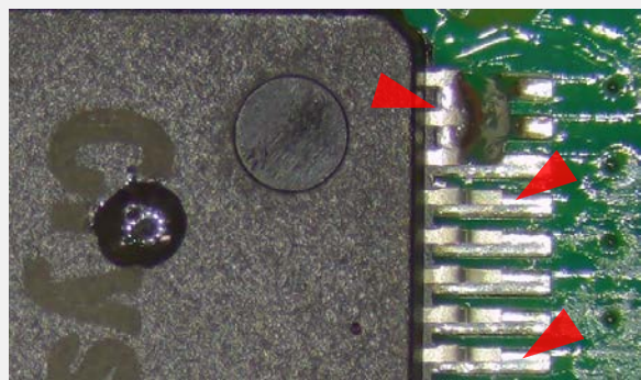
はんだブリッジ&はんだ不足 IPC-A-610G 5.2.7.2, 8.3.5を参照
