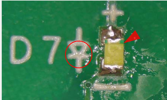
取付方向相違 IPC-A-610G 7.1.1.1を参照
