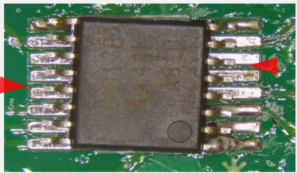
リードサイドのはみ出し&はんだ不足 IPC-A-610G 8.3.5を参照
