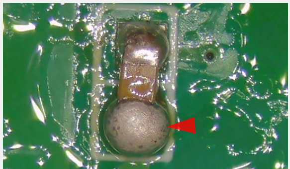
はんだ過多 IPC-A-610G 8.3.2を参照
