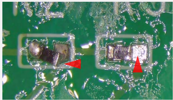
サイドのはみ出し&はんだ不足 IPC-A-610G 8.3.2を参照
