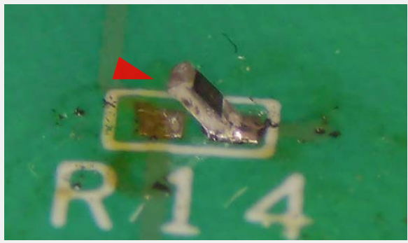
ズームストーン現象 IPC-A-610G 8.3.2.9.4を参照
