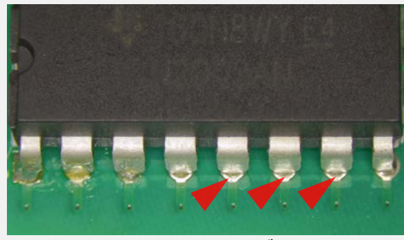
リードとスルーホール間のはんだのぬれ不足 IPC-A-610G 7.3.5を参照
