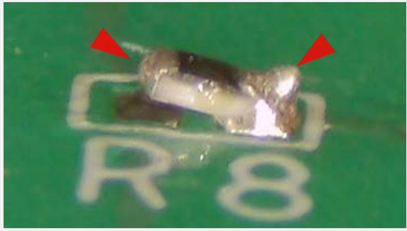
ズームストーン現象&はんだの突起 IPC-A-610G 8.3.2.9.4, 5.2.10を参照
