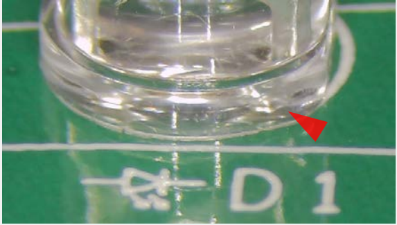
ラジアルリード垂直方向 クリアランス不足 IPC-A-610G 7.1.6を参照
