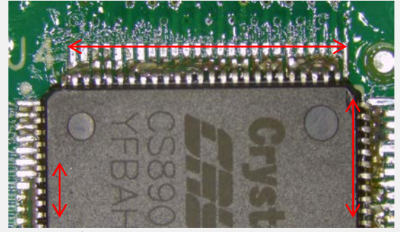
はんだブリッジ IPC-A-610G 5.2.7.2を参照
