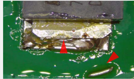
コールドはんだ接合&FOD IPC-A-610G 5.2.5, 10.6.2を参照
