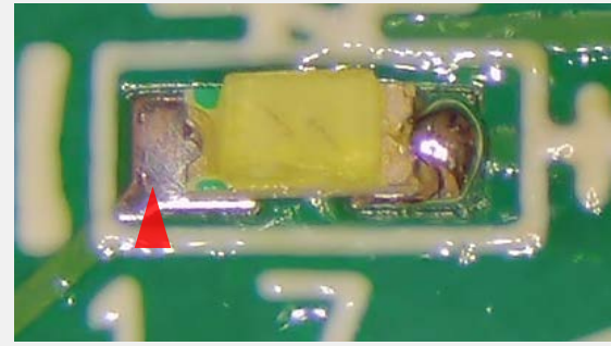
はんだ不足 IPC-A-610G 8.3.2を参照
