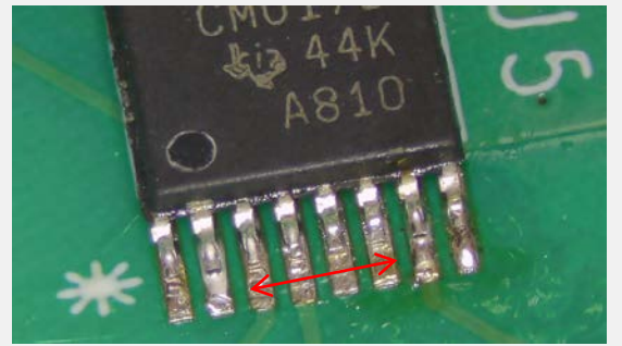
はんだ不足 IPC-A-610G 8.3.5を参照
