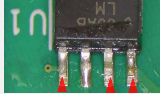
はんだ不足 IPC-A-610G 8.3.5を参照
