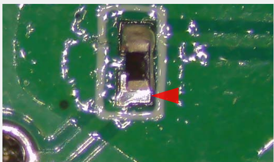
はんだ不足 IPC-A-610G 8.3.2を参照
