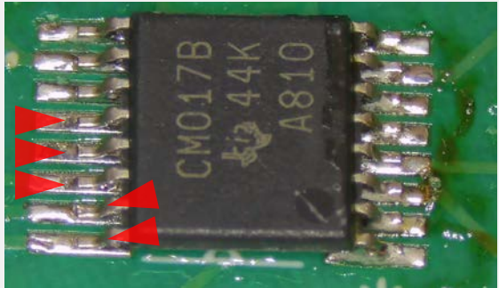
はんだ不足 IPC-A-610G 8.3.5を参照
