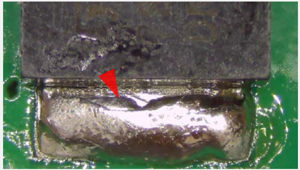
コールドはんだ接合 IPC-A-610G 5.2.5を参照
