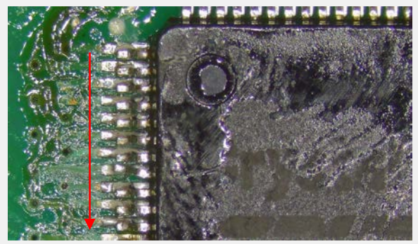
リードサイドのはみ出し IPC-A-610G 8.3.5を参照
