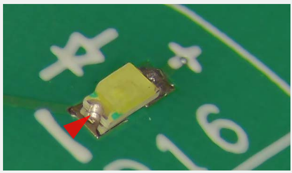
はんだ不足 IPC-A-610G 8.3.2を参照
