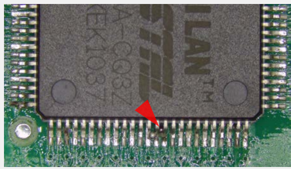
はんだブリッジ IPC-A-610G 5.2.7.2を参照
