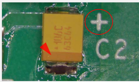
取付方向相違 IPC-A-610G 7.1.1.1を参照
