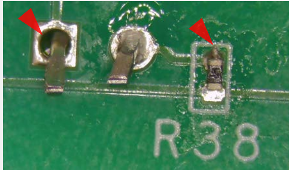
はんだ不足&はんだの突起 IPC-A-610G 7.3.5, 5.2.10を参照
