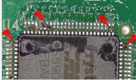
はんだブリッジ IPC-A-610G 5.2.7.2を参照
